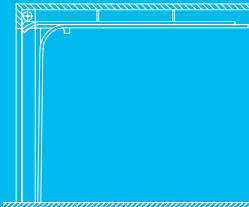
Prowadzenie typu LHRF Niskie – ze sprężynami z przodu
