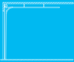
Prowadzenie typu NP Normalne
