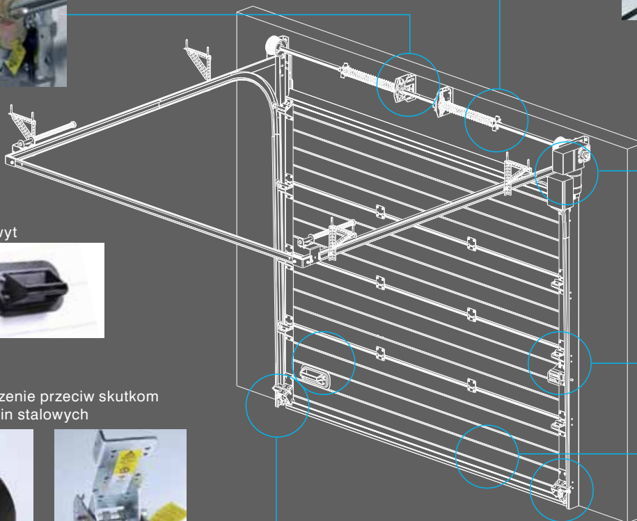
Zabezpieczenie przeciw skutkom pęknięcia sprężyn
